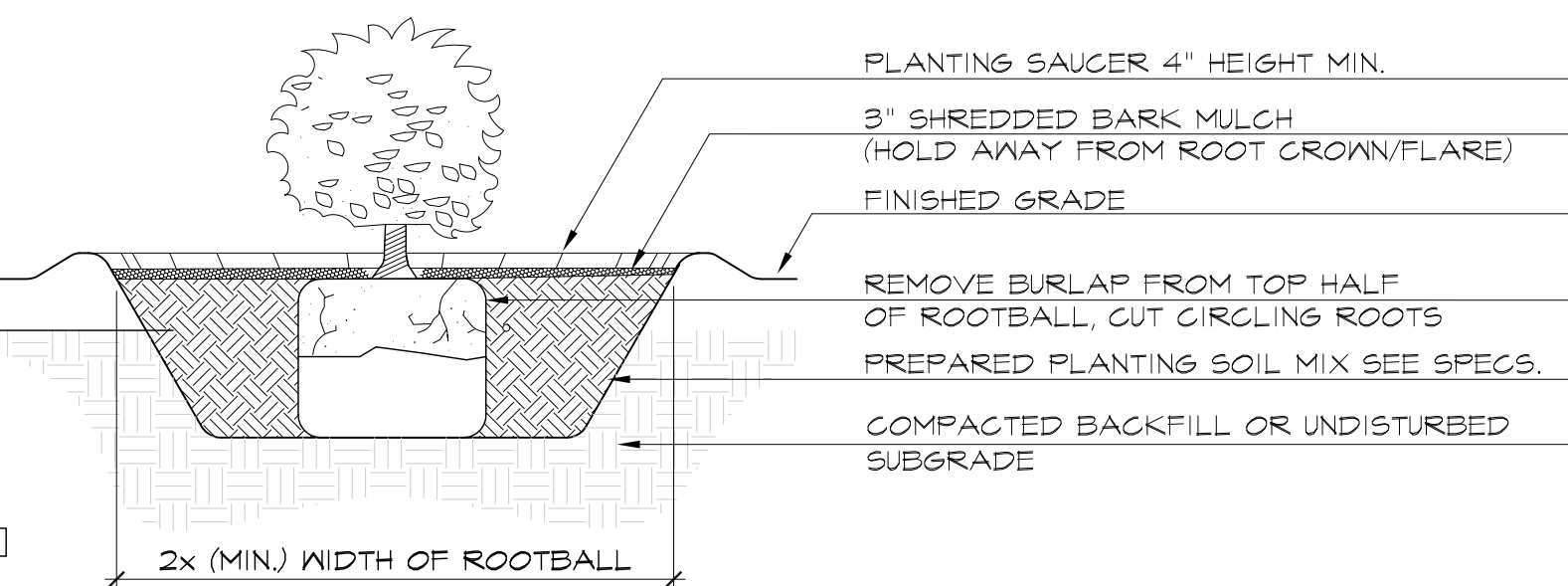
4 SHRUB PLANTING SCALE: N.T.S.
